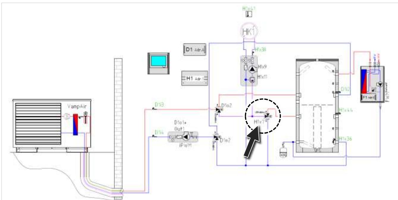
Abb. 9-12 – Kühlventil am Ausgang x7 des Elektronikmoduls H1
