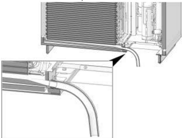
Abb. 5-3: K 08, K 10 – Ablauf nach unten
