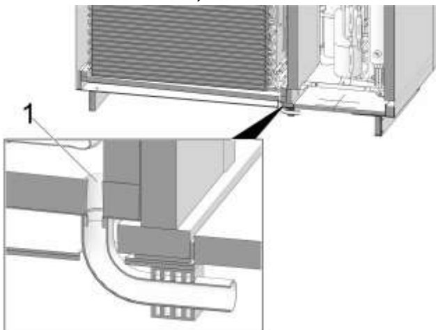
Abb. 5-4: K 12, K 15 – Ablauf seitlich
