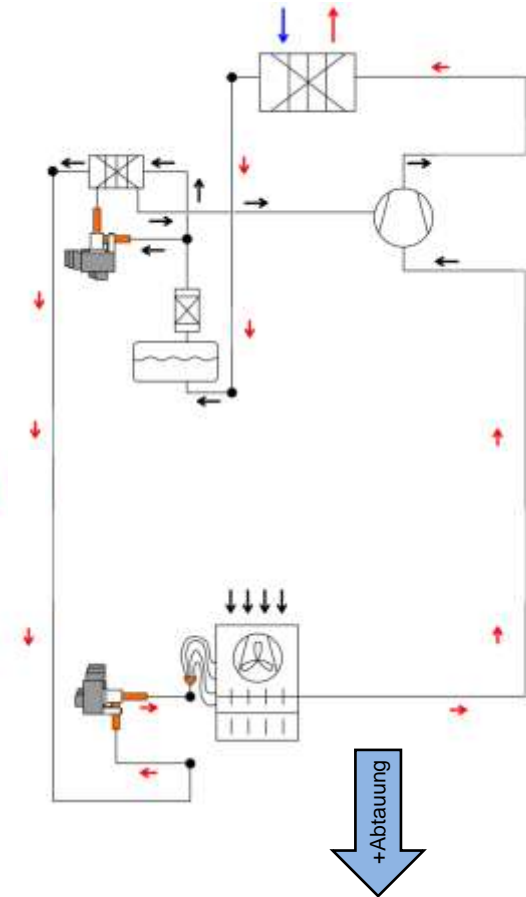
Kreisprozess mit Abtauung und mit EVI (=vamp air )
