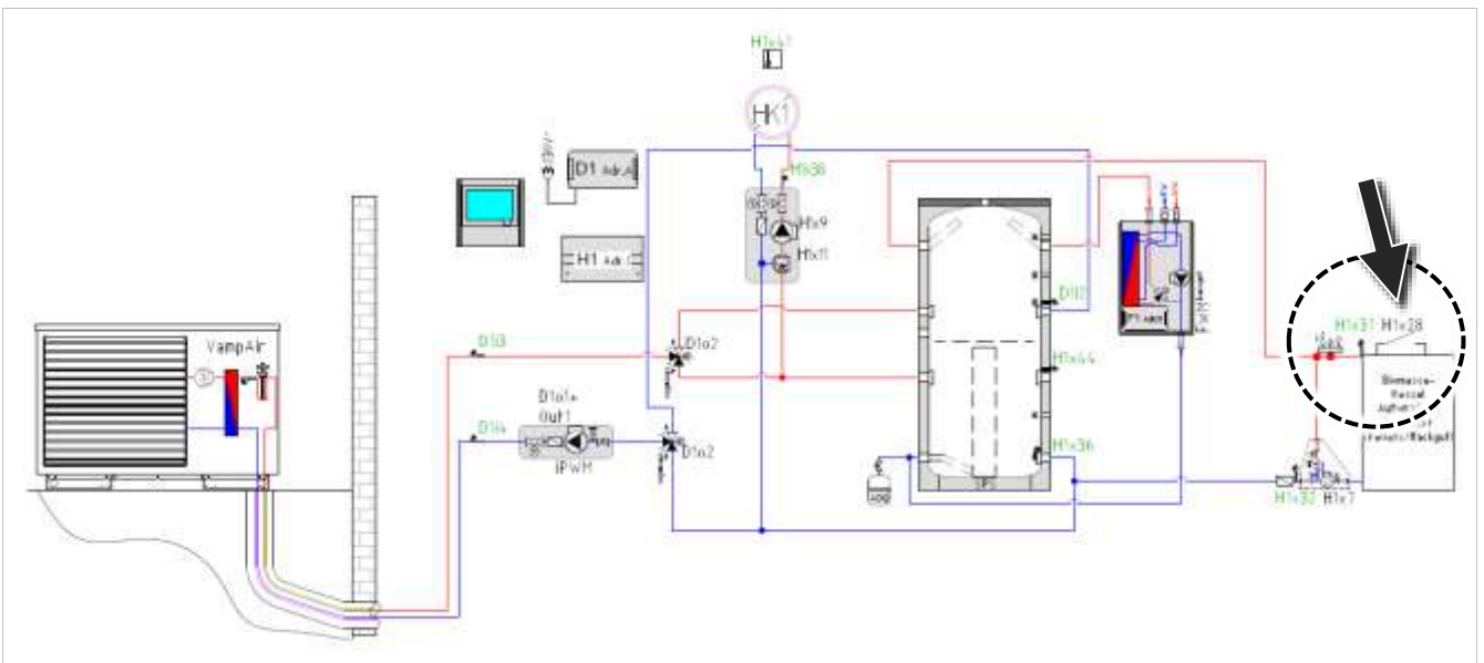
Abb. 9-17 – Relaisausgang X28 am Elektronikmodul H1
