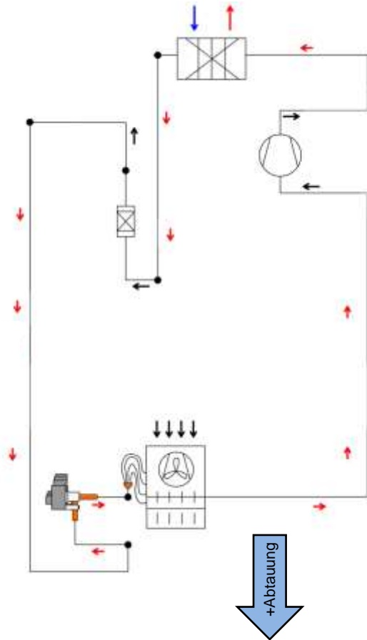
Kreisprozess mit Abtauung
