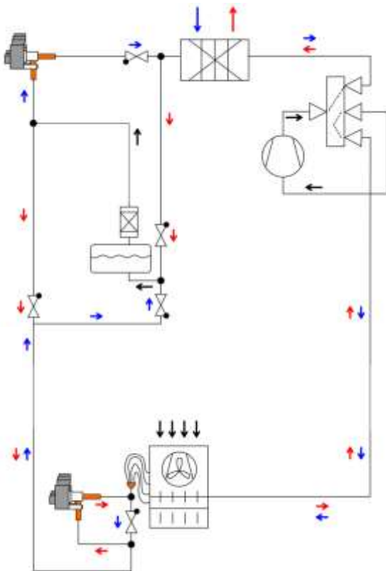
Kreisprozess mit Abtauung
