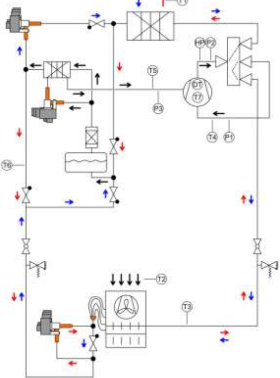
Kreisprozess mit Abtauung und mit EVI (=vamp air )
