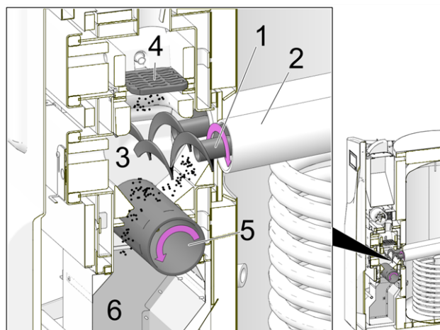
Abb. 2-49: Coupe du brûleur
