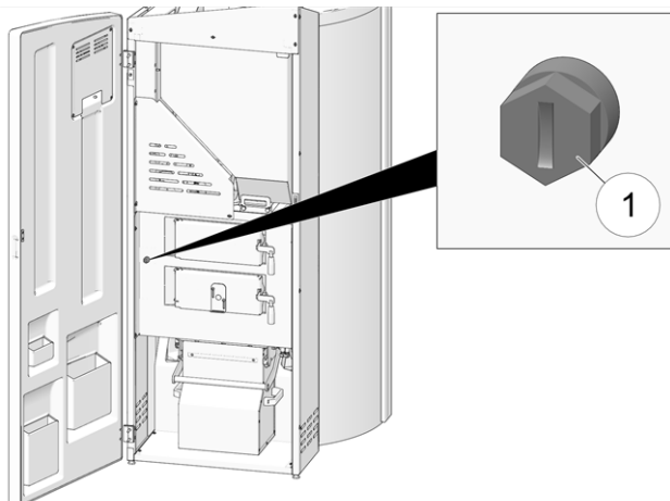
Abb. 2-1: Position du LTS
