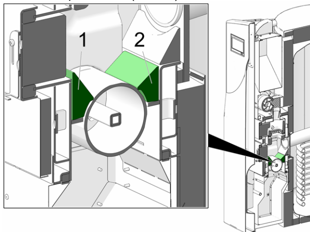
Abb. 2-55: Disposition des briques réfractaires dans la chambre de combustion
