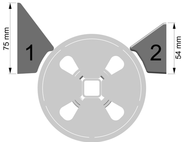
Abb. 2-56: Différence de hauteur des briques réfractaires
