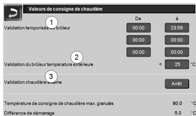
Abb. 2-8: Valeurs de consigne de la chaudière
