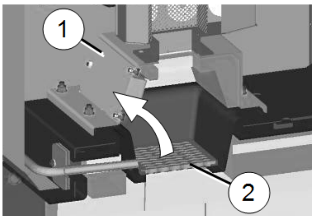
Abb. 2-56: Sostituire la griglia di combustione
