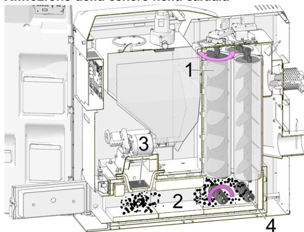
Abb. 2-51: Sezione della caldaia
