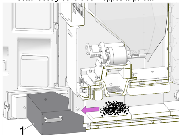
Abb. 2-54: Estrarre la cenere dalla camera di combustione nel cassetto raccogli cenere
